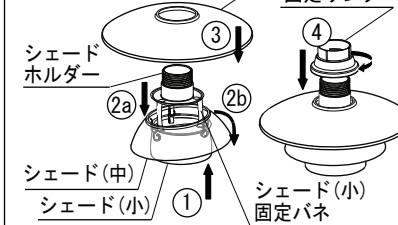
図2 シェードホルダーの取り付け
