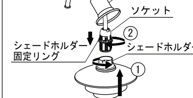
図3 ソケットカバーの取り付け
