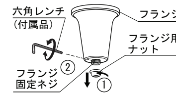
図1 フランジの取り付け方法
